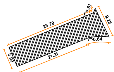
Detalhe 1 - área de fresagem - 170,56m 2
