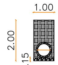
Área de Aterro = 1,39m² TUBO DN=600mm
