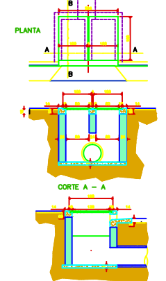
Boca de Lobo Dupla c/ Tapa de Concreto
