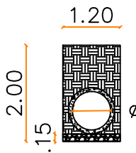
Área de Aterro = 1,49m² TUBO DN=800mm
