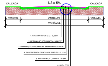
RUA JAÇANÃ TRECHO 01 E RUA JACUMÃ SEÇÃO TRANSVERSAL PAVIMENTAÇÃO ASFÁLTICA
