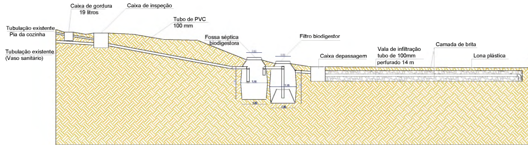
Implantação típica Escala: 1:40
