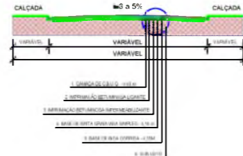
RUA JAÇANÃ TRECHO 01 E RUA JACUMÃ SEÇÃO TRANSVERSAL PAVIMENTAÇÃO ASFÁLTICA
