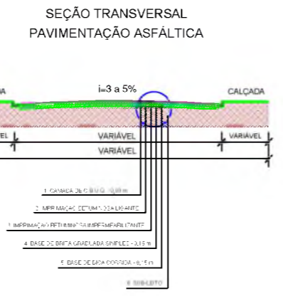
ALAMEDA JAÇANÃ- TRECHO 02
