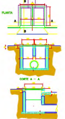
Boca de Lobo Dupla c/ Tampa de Concreto
