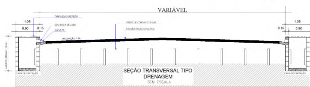
DETALHAE- REDE DE DRENAGEM - S/ESC
