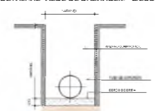
DETALHAE- REDE DE DRENAGEM - S/ESC
